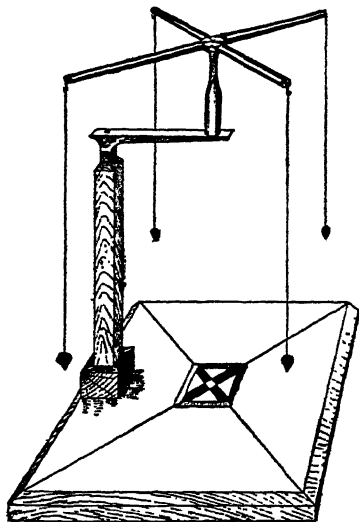
FIG. 49. The Groma.
