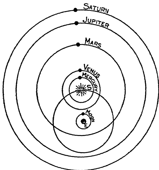
FIG. 56. Tycho's World-System.
