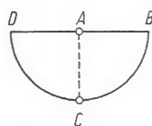
Velocity plane ( \bar{w} -plane)
