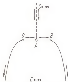
Stream plane ( z -plane)
